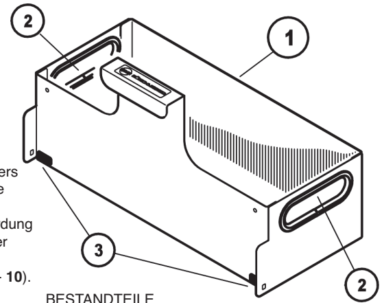
BESTANDTEILE
