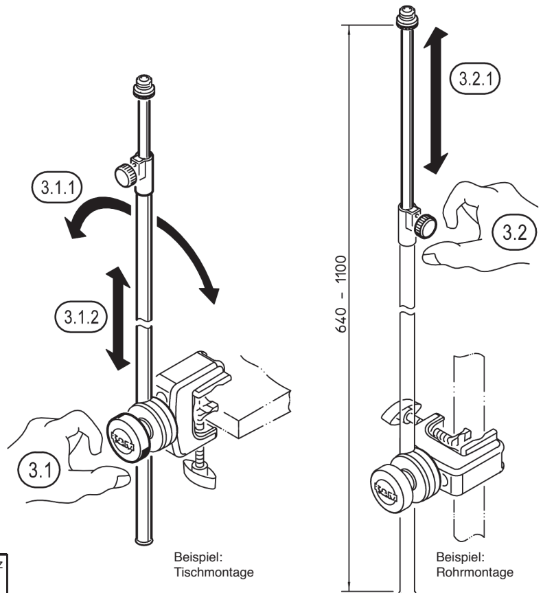
1. BESTANDTEILE und MONTAGE
