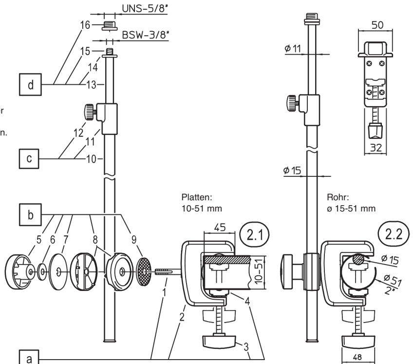
1. BESTANDTEILE und MONTAGE
