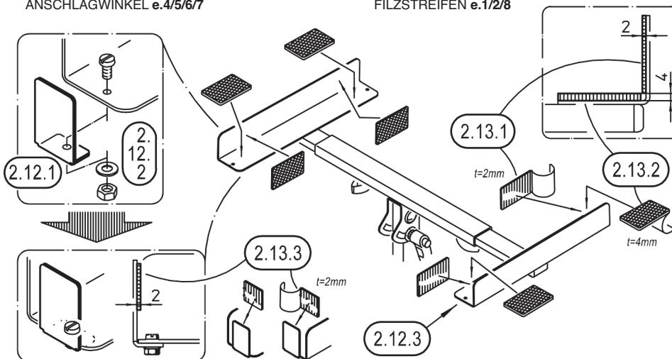
ANSCHLAGWINKEL e.4/5/6/7
