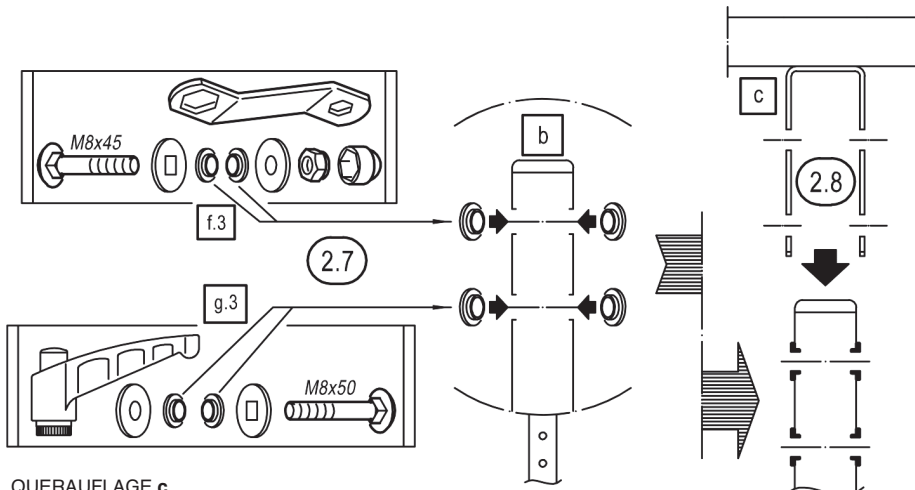
QUERAUFLAGE c
