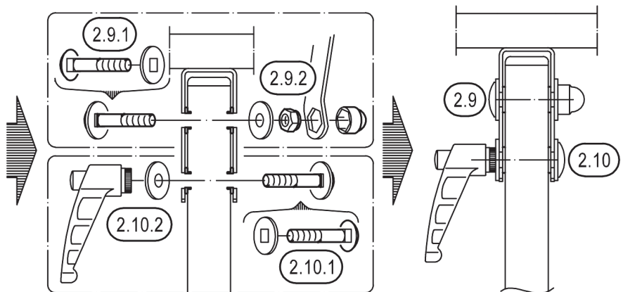
VERSTELLBÜGEL d, e.3
